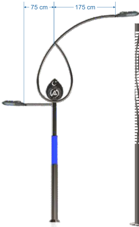
EL-98.1426 h:700 cm Çelik Boru Armatür dahil değildir
