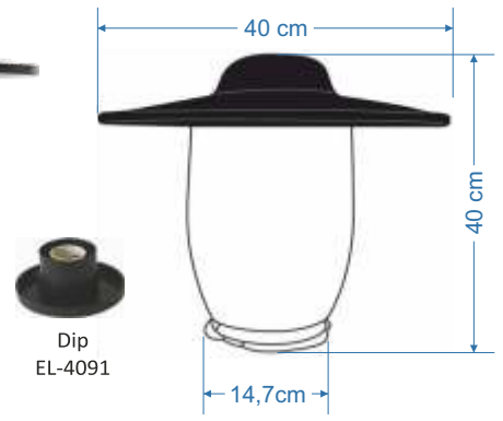
EL-4080 Ø40 Uarus Şeffaf PMMA Tırnaklı Glop Koli Adeti: 5
