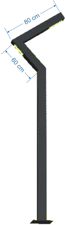
EL-98.1420 h:300 cm Çelik Profil Akıllık Cam 2x40W Led
