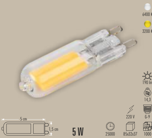
CT-4221 COB LEDLİ G-9 KAPSÜL 220 V
