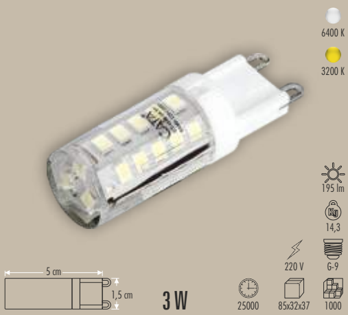
CT-4249 LEDLİ G-9 KAPSÜL 220 V
