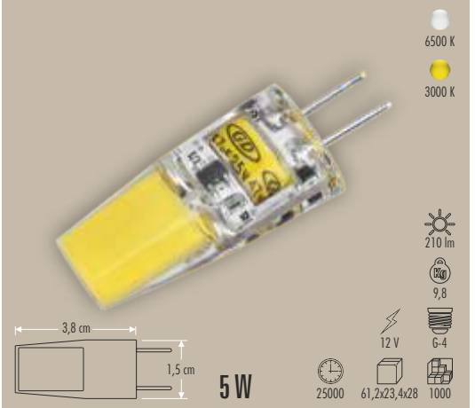
CT-4252 COB LEDLİ G-4 KAPSÜL 12 V
