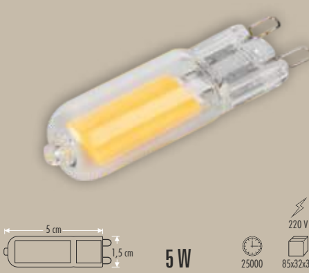
CT-4221 COB LEDLİ G-9 KAPSÜL 220 V
