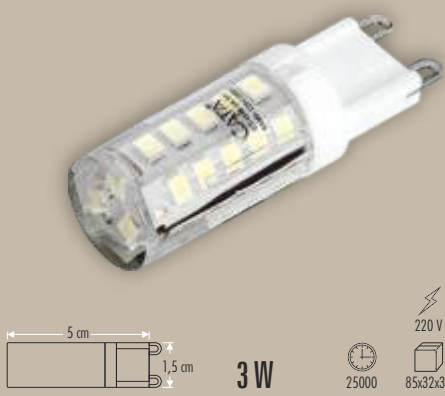
CT-4249 LEDLİ G-9 KAPSÜL 220 V
