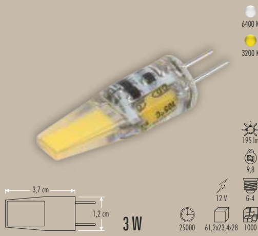
CT-4255 COB LEDLİ G-4 KAPSÜL 12 V
