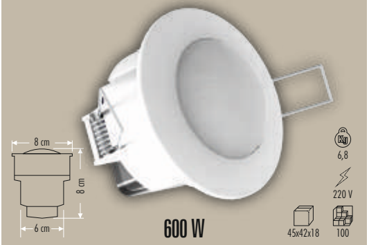
CT-9242 SIVA ALTI SENSÖR
